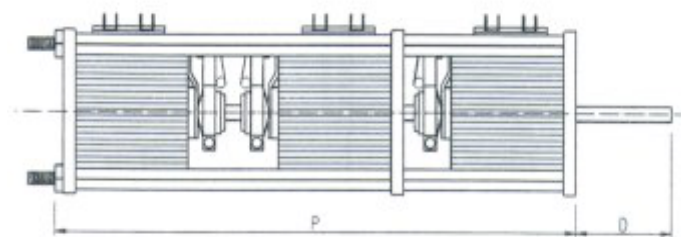
MISURE DI INGOMBRO (mm)
